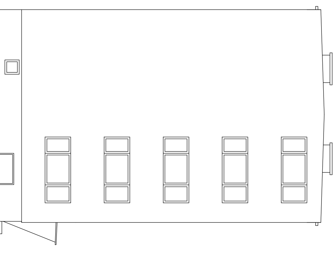
ELEWACJA WSCHODNIA
